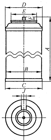
图 B.1 气瓶
