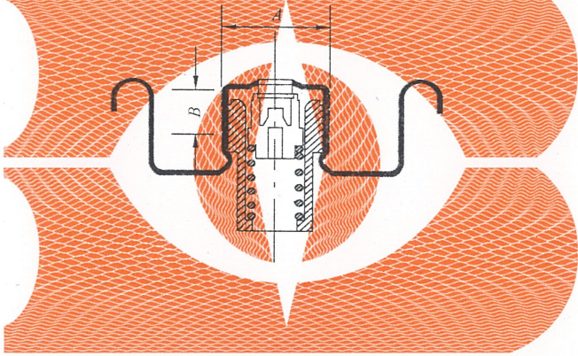
图 B.3 高山气瓶阀门公螺纹接口示意图
